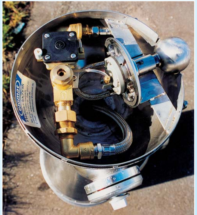
Das Innenleben des Pepino Trinkbrunnen mit Zeitglied und Verrohrtechnik.
